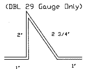
Snow Bar
